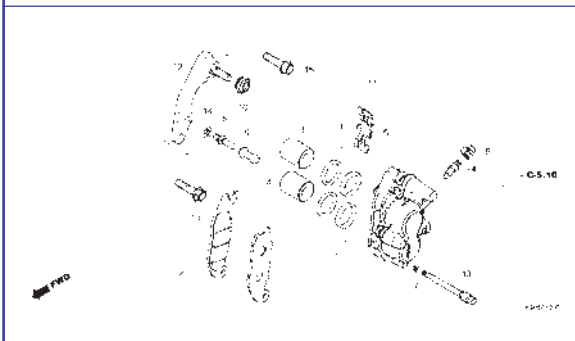
C-17 Cáliper do Freio Traseiro
