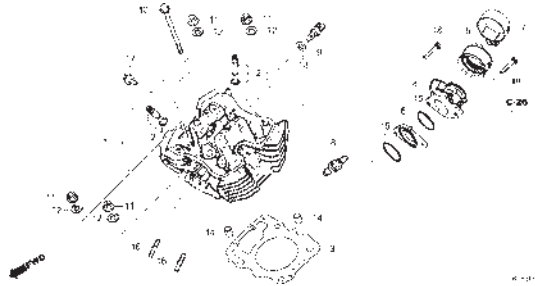
M-5 Cilindro
