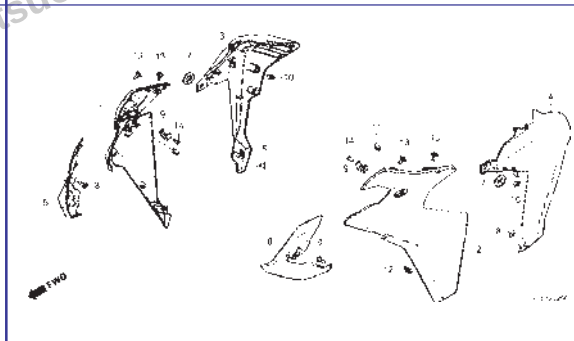
C-22 Carenagem
